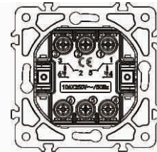
Выключатель двухклавишный проходной (на 2 направления) с подсветкой
